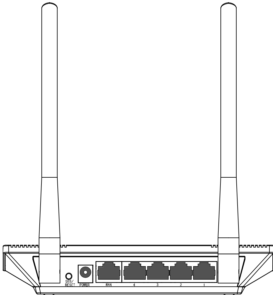
图 3-2 TL-WR845N 后面板示意图
