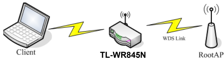
图 5-12 WDS 连接拓扑图
