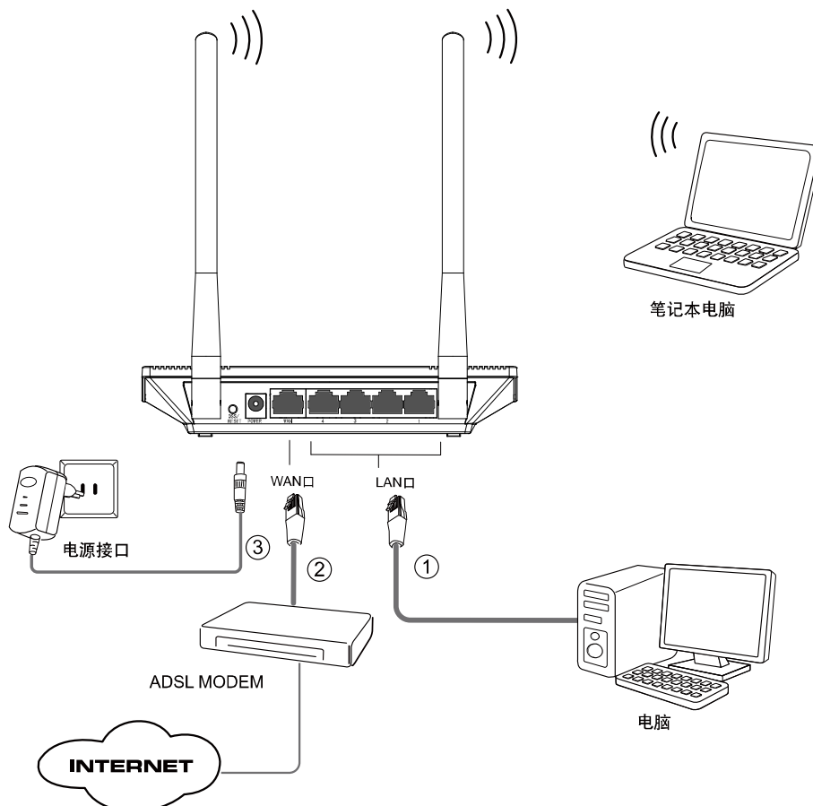
图 4-1 TL-WR845N 硬件安装示意图
